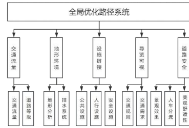
图 6：全局优化路径系统策略图
